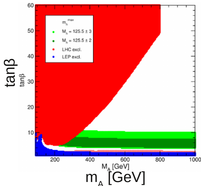
“mh-max” scenario
