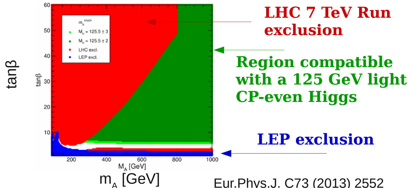
“mh-mod+” scenario
